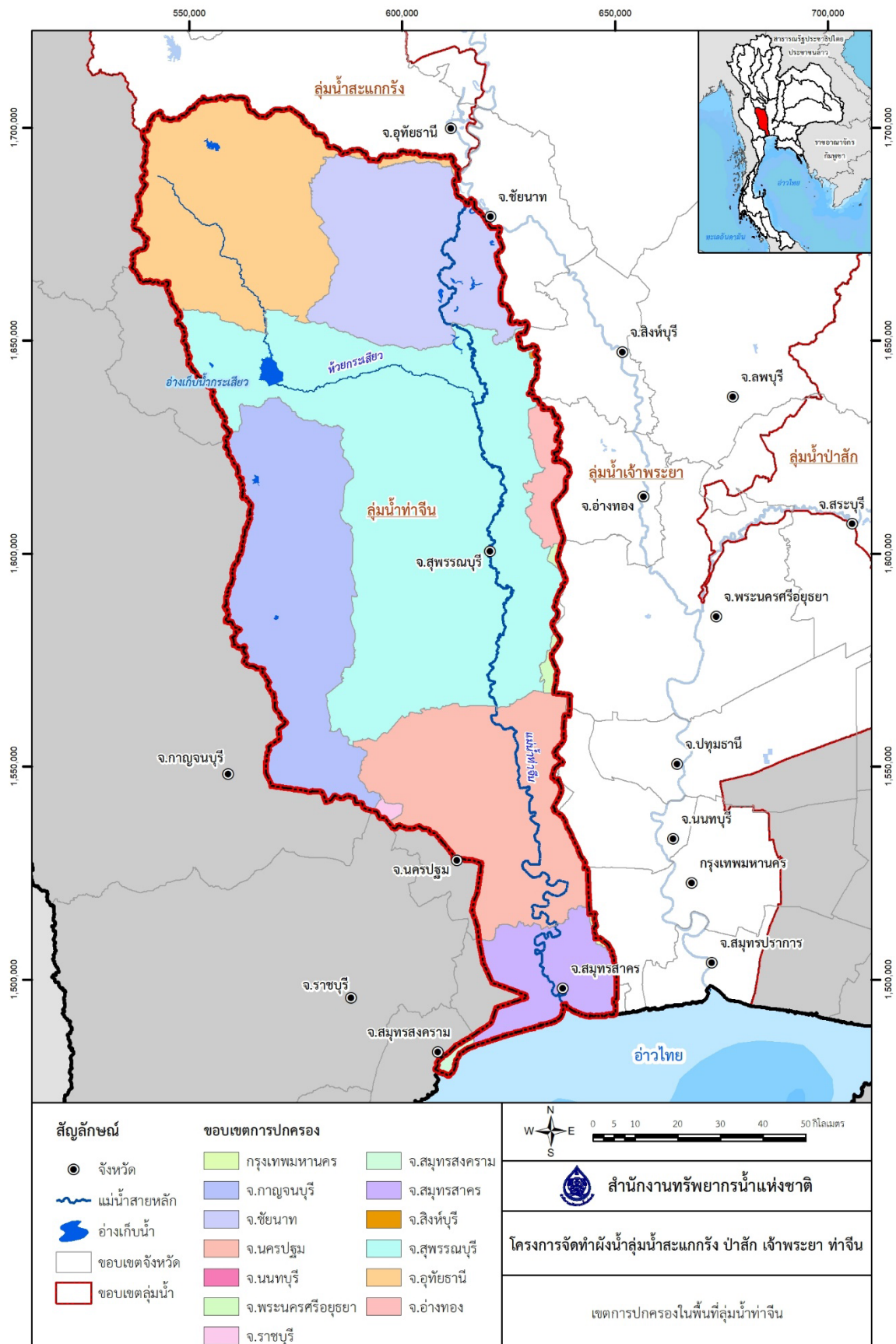
รูปที่ 2.3-1 เขตการปกครองในพื้นที่ลุ่มน้ำท่าจีน
