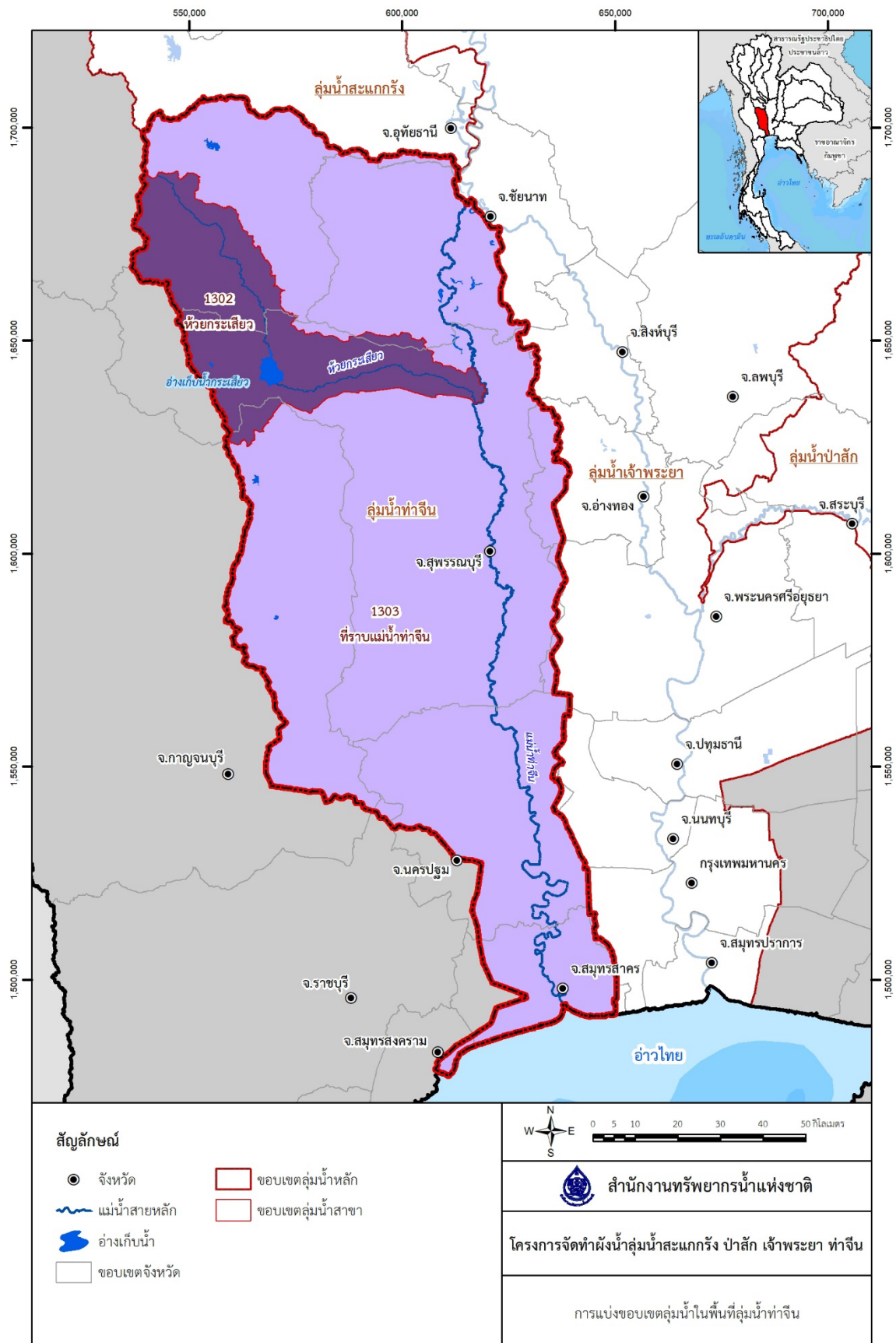
รูปที่ 2.2-1 การแบ่งขอบเขตลุ่มน้ำในพื้นที่ลุ่มน้ำท่าจีน
