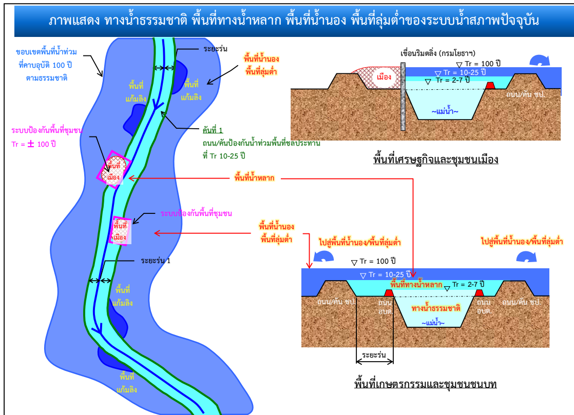
รูปที่ 3.4-1 (ข) ทางน้ำธรรมชาติ พื้นที่ทางน้ำหลาก พื้นที่น้ำนอง พื้นที่ลุ่มต่ำของสภาพปัจจุบัน
