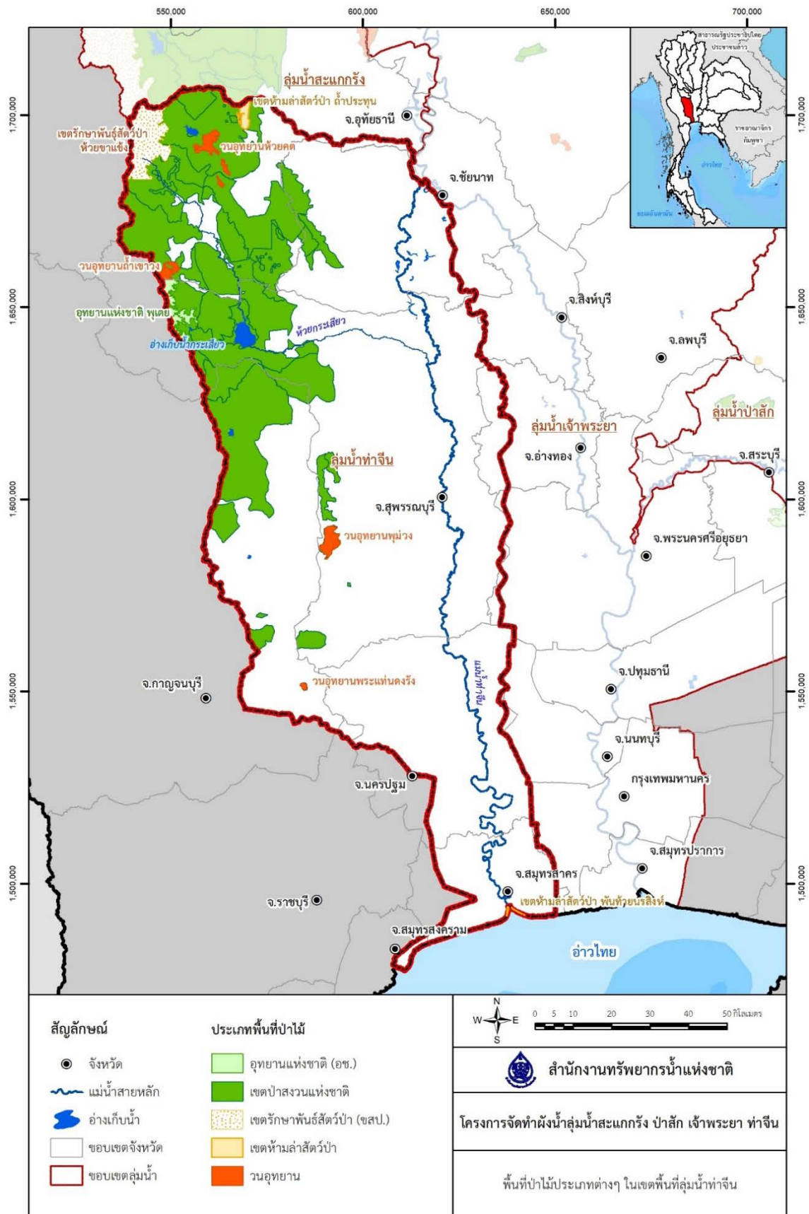
รูปที่ 2.6-1 พื้นที่ป่าไม้ประเภทต่าง ๆ ในเขตพื้นที่ลุ่มน้ำท่าจีน
