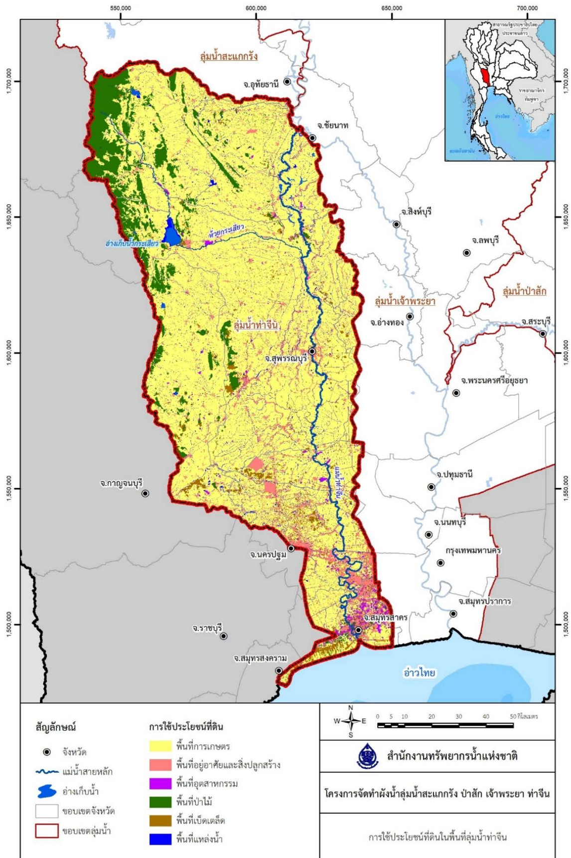
รูปที่ 2.7-1 การใช้ประโยชน์ที่ดินในพื้นที่ลุ่มน้ำท่าจีน
