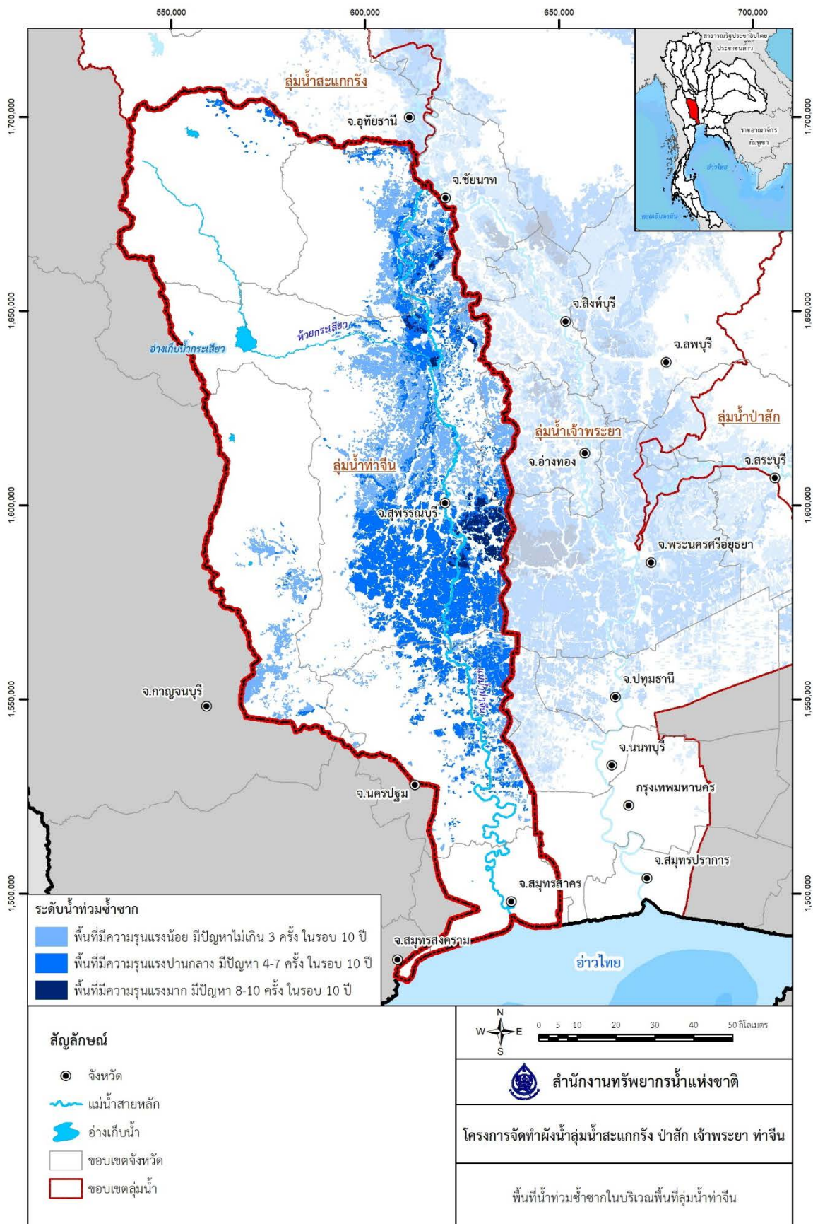
รูปที่ 2.11-1 พื้นที่ประสบปัญหาน้ำท่วมซ้ำซากในลุ่มน้ำท่าจีน
