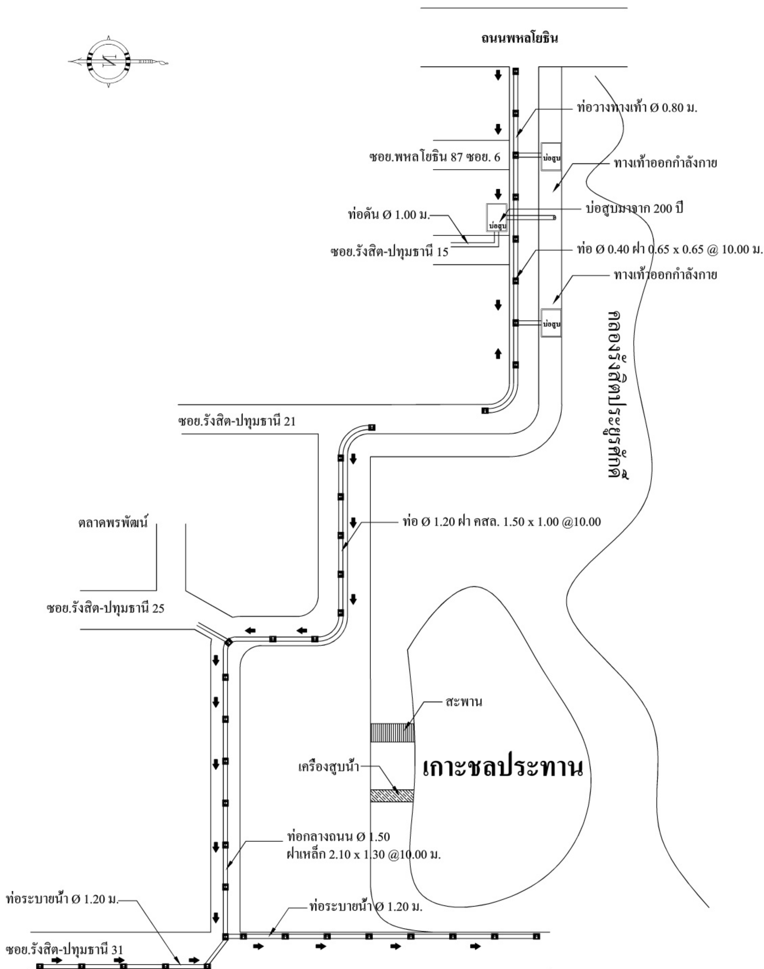
14 ผังระบบท่อระบายน้ำ ถนนพหลโยธิน 127 ( เลียบคลองฝั่งเหนือ )
